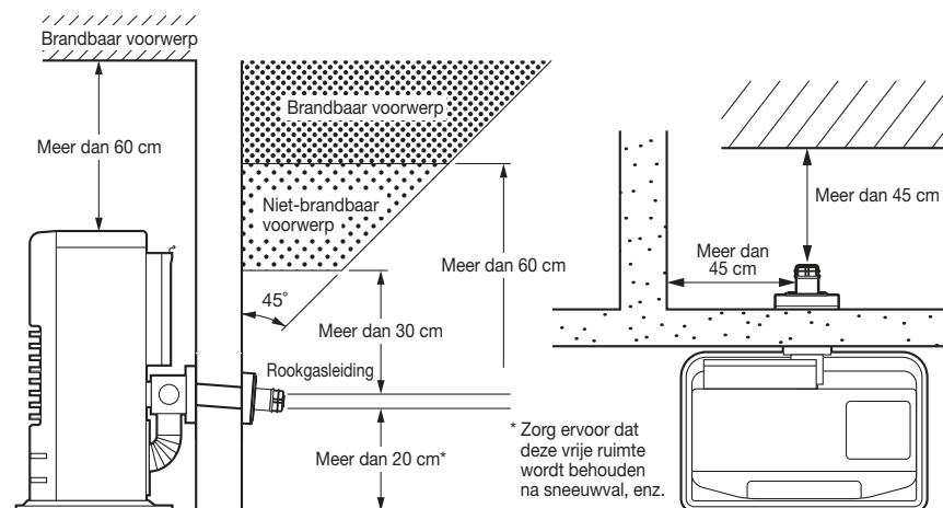
Afb. 2 Installatie van de rookgasleiding
